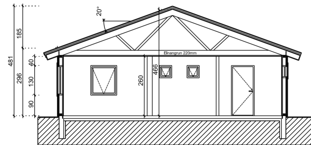
Snið C-C 1:100
