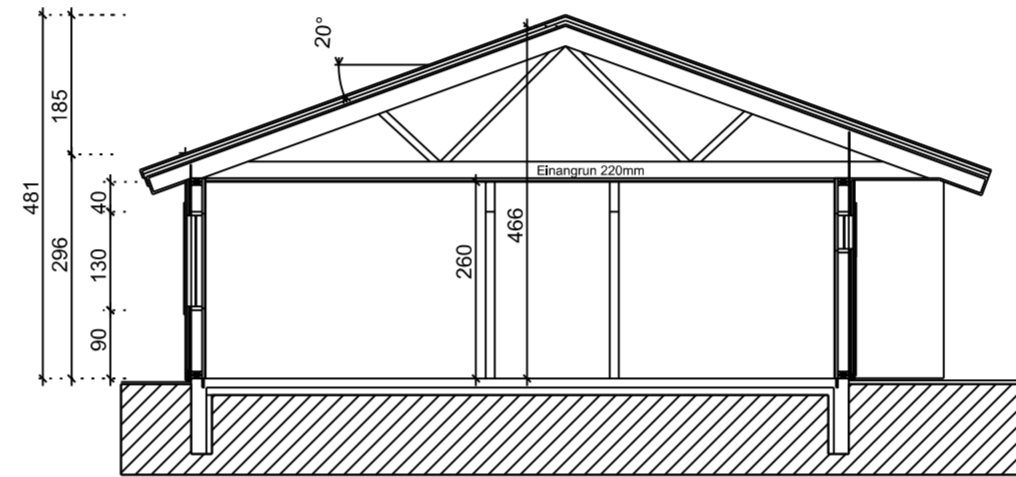
Snið B-B 1:100
