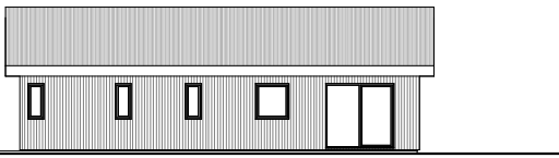
Suður 1 : 100
