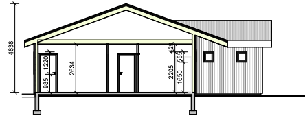
Snið A 1 : 100
