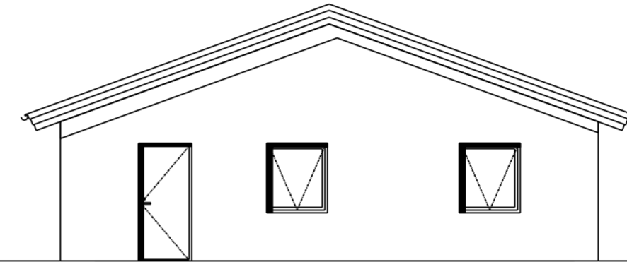
Norðurhlíð 1:100
