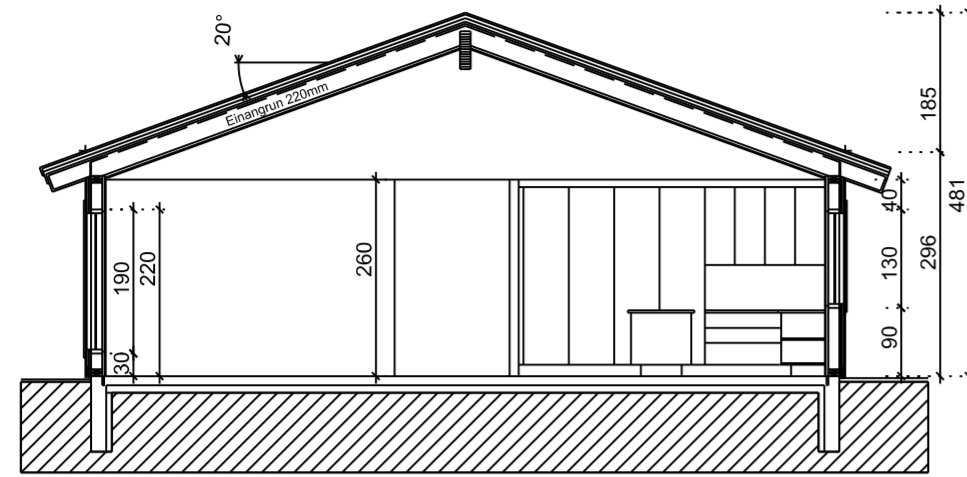
Snið A-A 1:100
