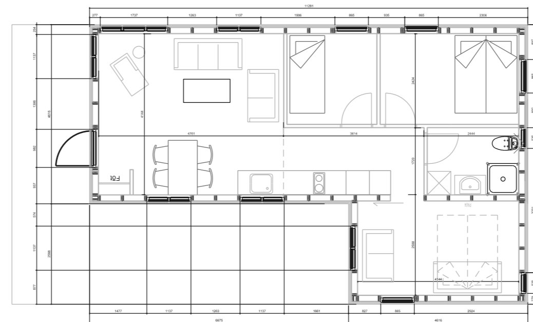
GRUNNMYND, 1:50
